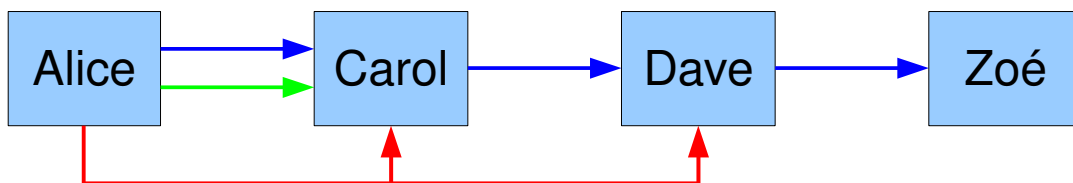
FIGURE 4 – Schéma de principe de la non-transitivité du réseau de confiance. La légende est celle de la figure 3. Alice a vérifié la clé de Carol et a confiance en elle, et celle-ci a vérifié la clé de Dave. Alice a donc une garantie de la validité de la clé de Dave, mais pas de celle de Zoé puisqu'Alice n'a pas confiance en Dave.
